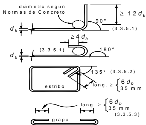
Figura 3.9 Dobleces del refuerzo
