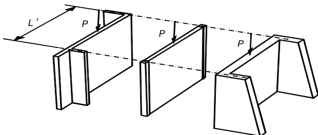
Figura 3.2 Restricción a la deformación lateral
