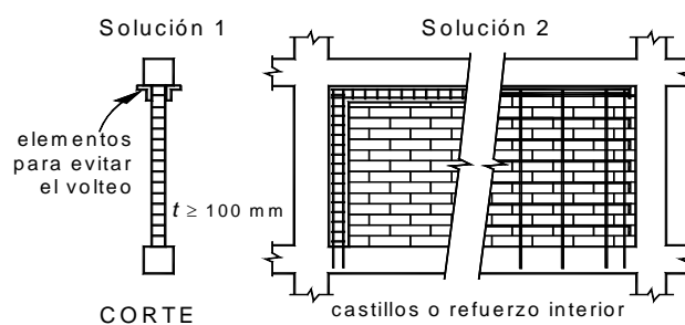
Figura 4.1 Detallado de muros diafragma
