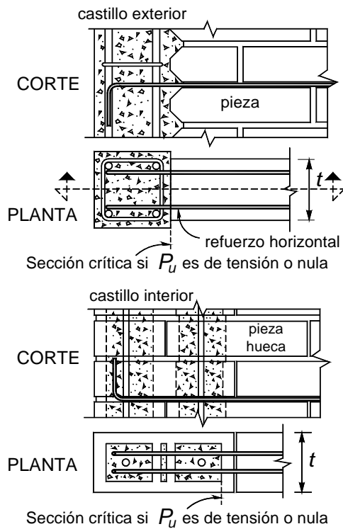
Figura 3.10 Anclaje de refuerzo horizontal
