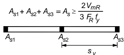
SECCIÓN DEL MURO
