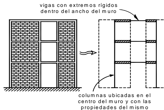
Figura 3.3 Modelo de columna ancha
