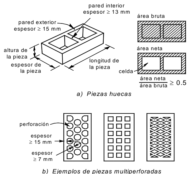
Figura 2.1 Piezas
