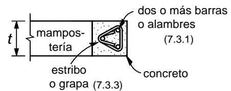
SECCIÓN DEL MURO
