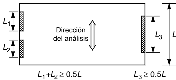
Figura 3.7 Requisito sobre muros de carga perimetrales paralelos
