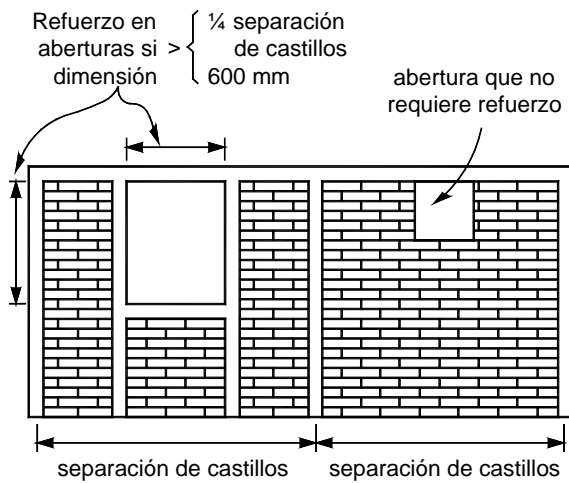
Figura 5.3 Refuerzo en el perímetro de aberturas
